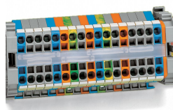
Bandes de marquage (709-196), sous lesquelles on distingue ici des peignes de pontage ;
