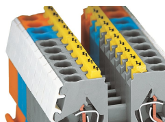
Obturbateur d'isolation, avec signalisation de danger (280-405)
