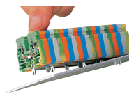
Barrette à bornes avec pieds de fixation, à encliqueter dans des trous
