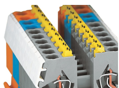
Obturateur d'isolation, avec signalisation de danger (280-405)
