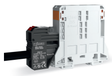
Montage via logement de pontage
