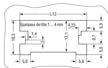
L12 = Nombre de pôles x pas + 10,2 mm
