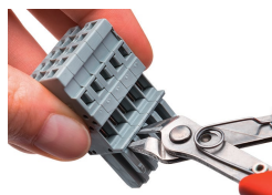
Kodierung einer Federleiste – Kodiernase (n) mittels Schneidwerkzeug entfernen. Die 1. und letzte Rastkodiernase nicht entfernen oder zusätzlich Verriegelungsklinke verwenden.
