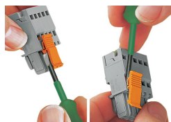
Verriegelungsklinke einrasten/lösen.
