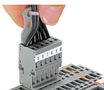
Herausziehen einer Federleiste am zugentlasteten Leiterbündel
