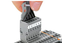
Herausziehen einer Federleiste am zugentlasteten Leiterbündel
