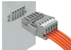
Stiftleiste und 1-Leiter-Federleiste mit seitlichen Verriegelungsklinken
