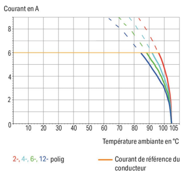
Courbe d'intensité maximale admissible Pas 2,5 mm / section de conducteur 0,5 mm 2 « s » Selon l'exemple de : EN 60512-5-2 / facteur de réduction 1
