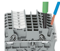
Leiter mit Betätigungswerkzeug anschließen.
